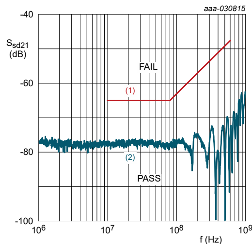
Fig. 20. Insertion loss
